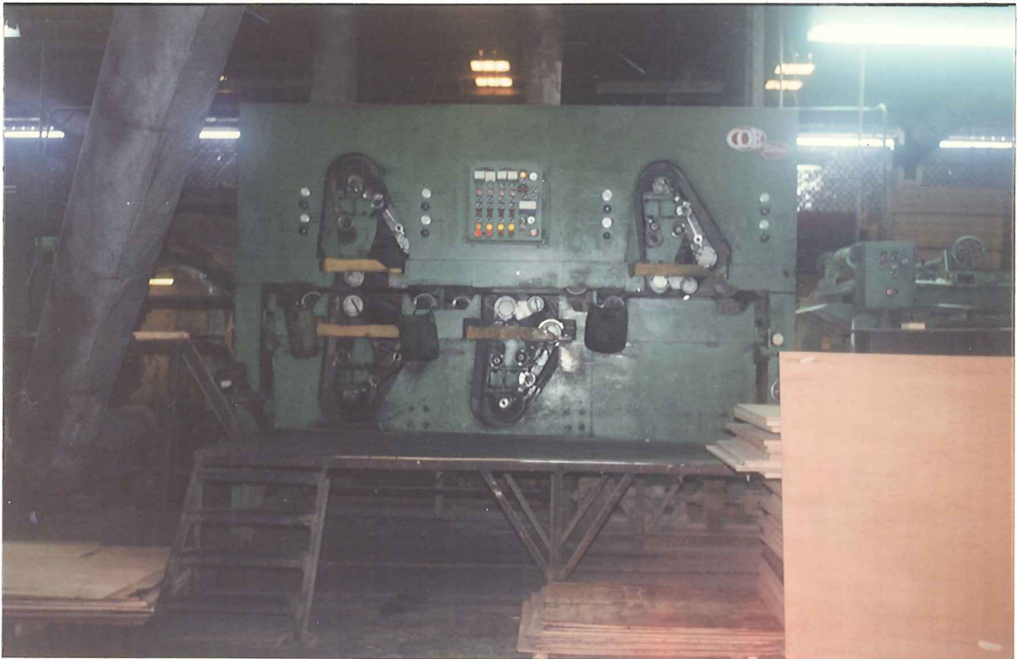
Foto nº 09 - Acabamento dos Compensados (Lixadeira) - AMAPLAC/Manaus
