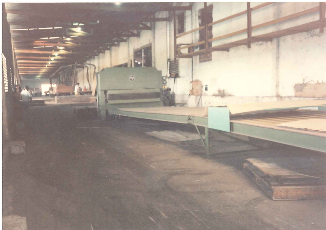
Foto nº 26 - Prensagem dos Compensados (Prensa)- KARSON/Xinguara
